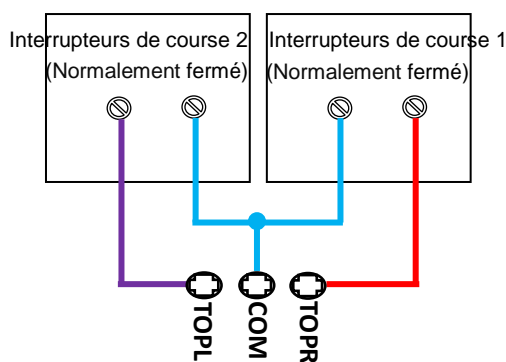
Connecter les Interrupteurs de course
